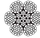
6xWS31+IWRC
